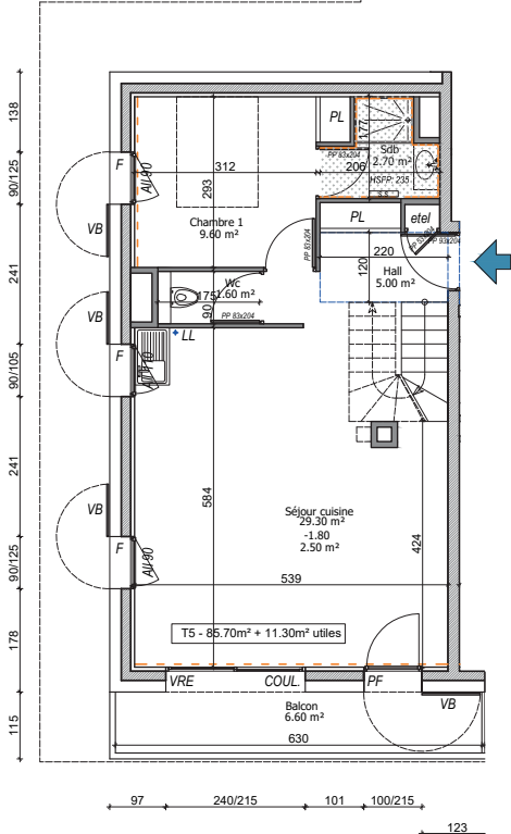
PLAN DU LOGEMENT NIVEAU R+1 ECH: 1 / 100
