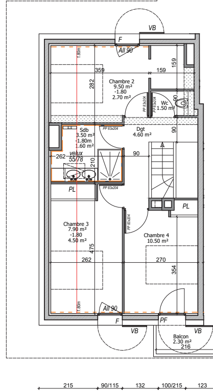
PLAN DU LOGEMENT NIVEAU R+2 ECH: 1 / 100
